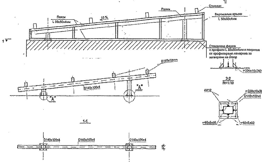
Ферми при крайни рамки за затваряне на отвори при едноскатен покрив
