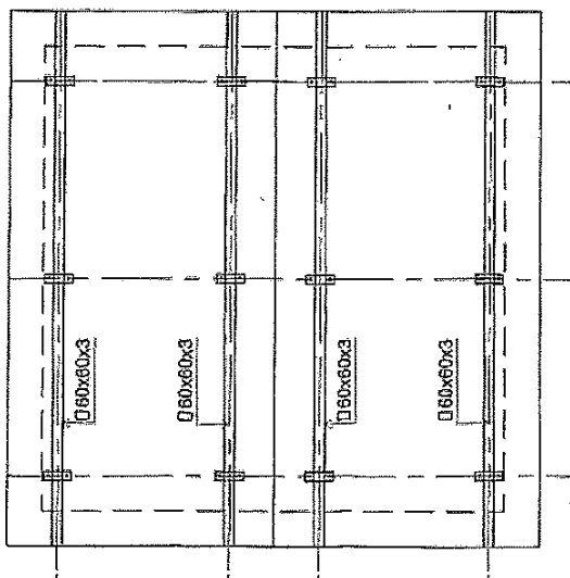
ПЛАН
