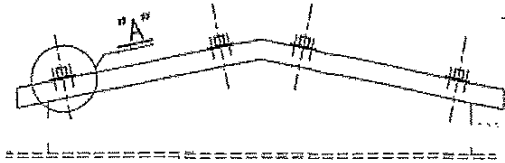
ПЛАН
